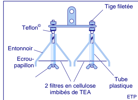
Capteur passif ETP
