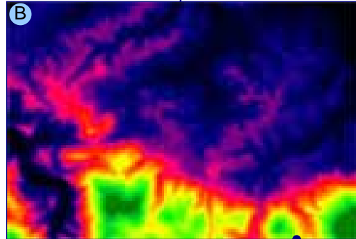
Biriadou - Carte des pentes
