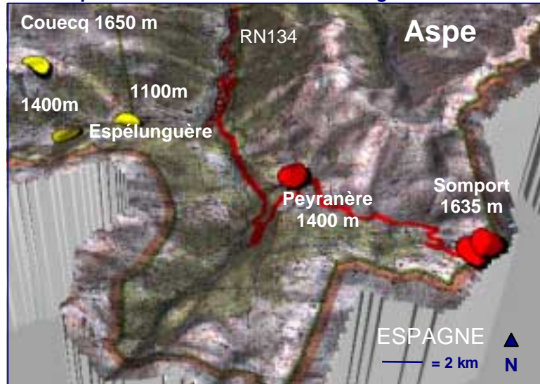
Sites de prélèvements des carottes de neige
