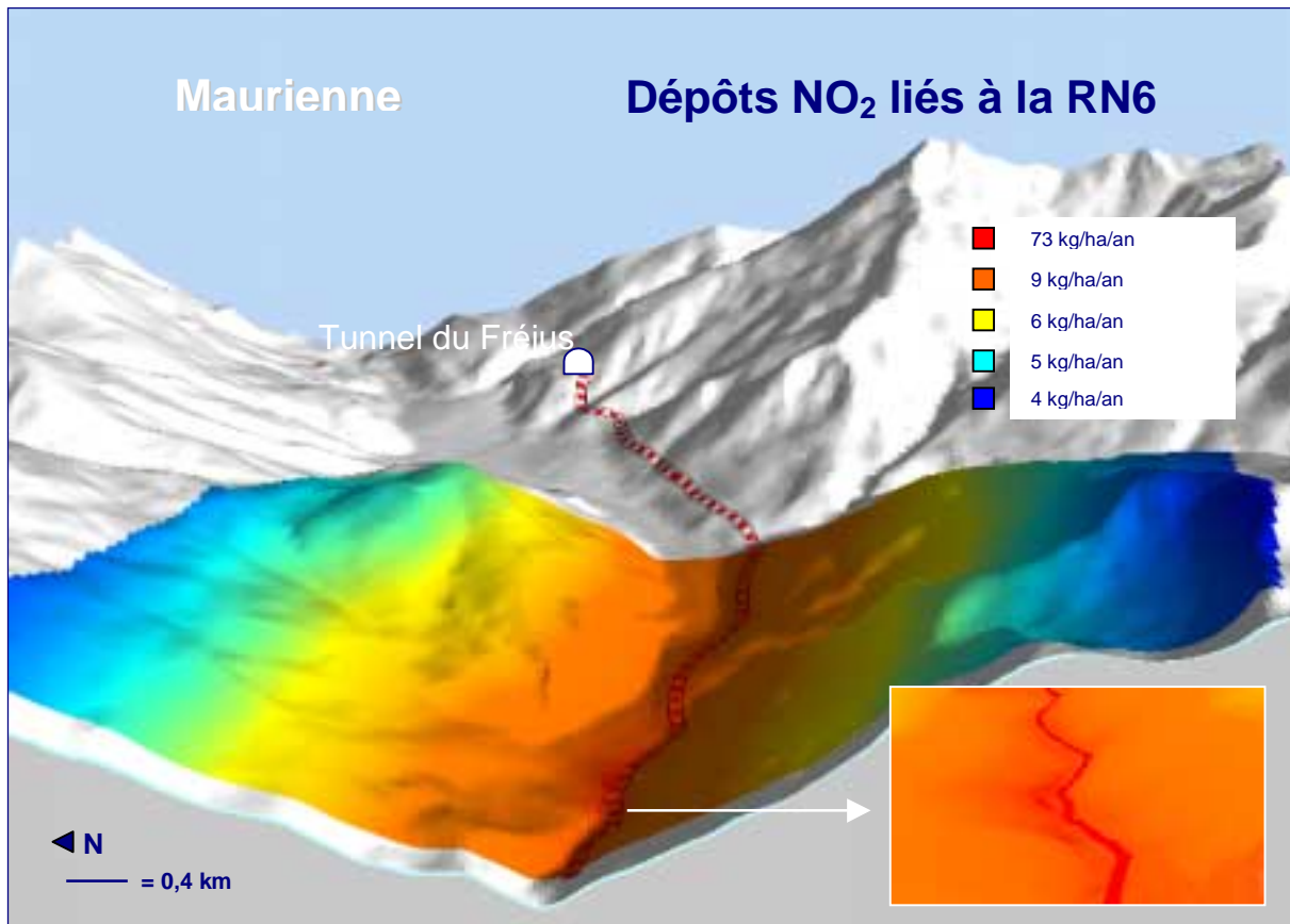
X : 939 000, Y : 2 030 930, azimuth : 270°, déclinaison : 25°, angle : 40, distance : 10 000 m
