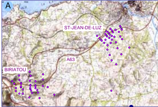
Biriadou - Emplacement des capteurs
