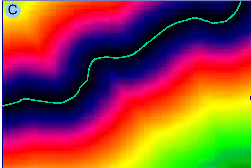
Biriadou - Fonction de décroissance du dépôt de NO 2
