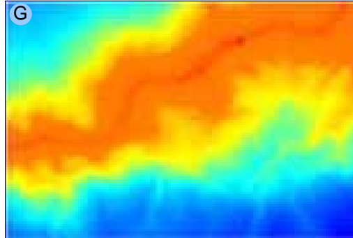
Biriadou - Carte des dépôts de NO 2
