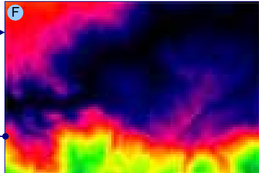
Biriadou - Carte des distances « réelles »
