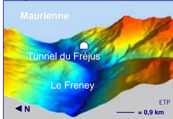
X : 939 000, Y : 2 030 930, azimuth : 270°, inclinaison : 25°, angle : 40, distance : 10 000
