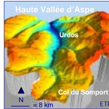
Configuration de l'altitude
